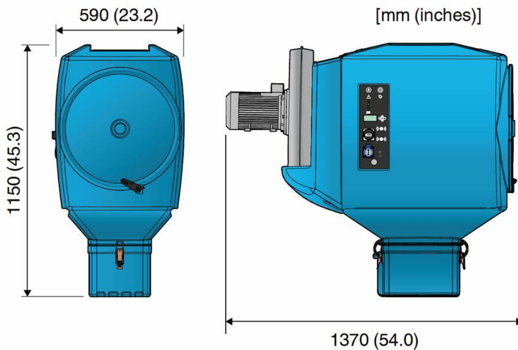
FilterBox nástěnná s N29 s ventilátorem
