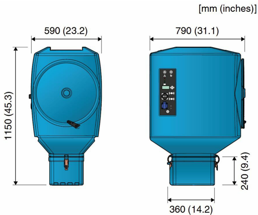
FilterBox nástěnná bez ventilátoru
