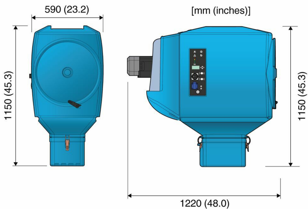
FilterBox nástěnná s N24
