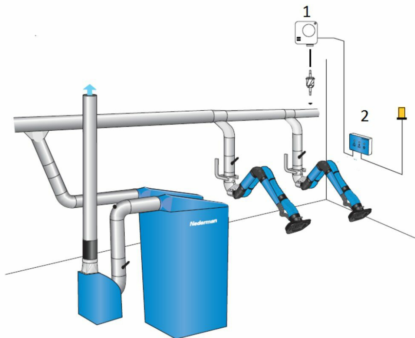
Alarm průtoku a montáž tlakového spínače 1) Tlakový spínač 2) Alarm průtoku
