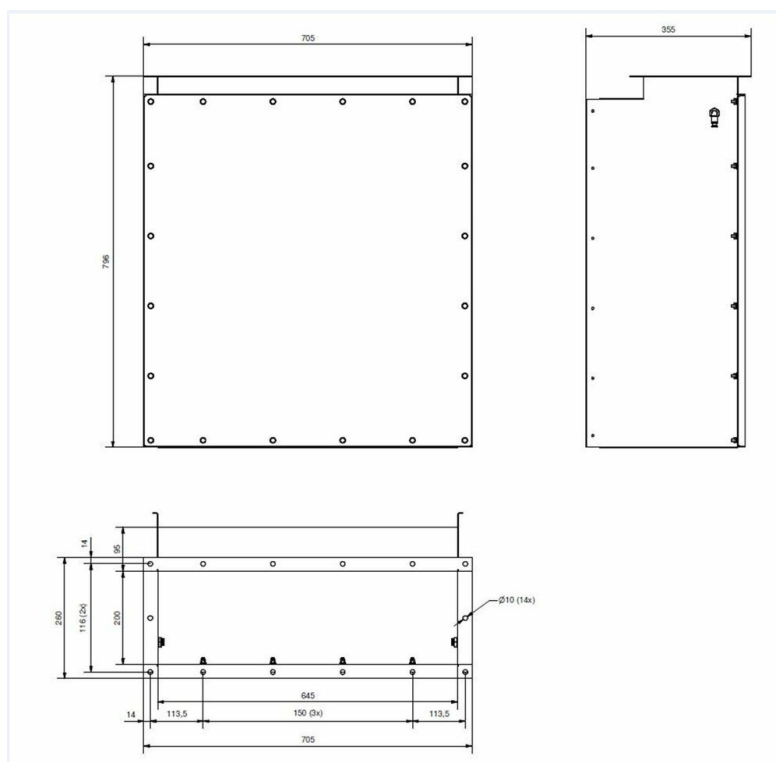
Výstupní připojení OSF 1000FC / OMF 2000FC - HEPA 610x610x150 mm
