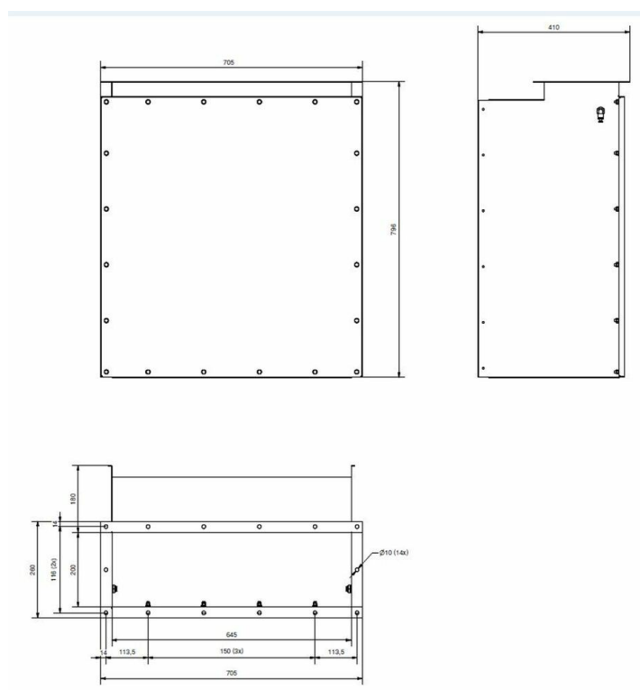
Výstupní připojení OSF 1000FC / OMF 2000FC - HEPA 610x610x292mm
