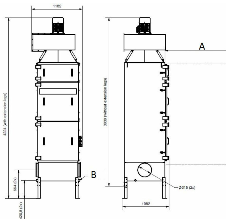
A) 1500 mm min servisní prostor B) výpust DN25 (2x)
