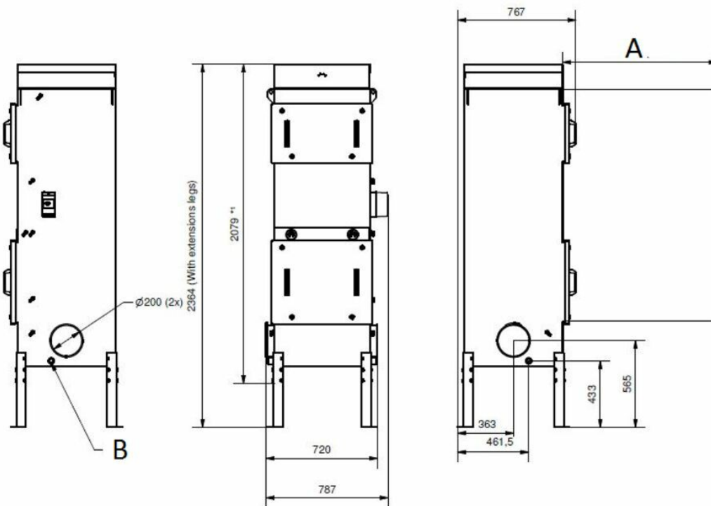
A) 1000 mm min servisní prostor B) Výpust DN25 (2x)
