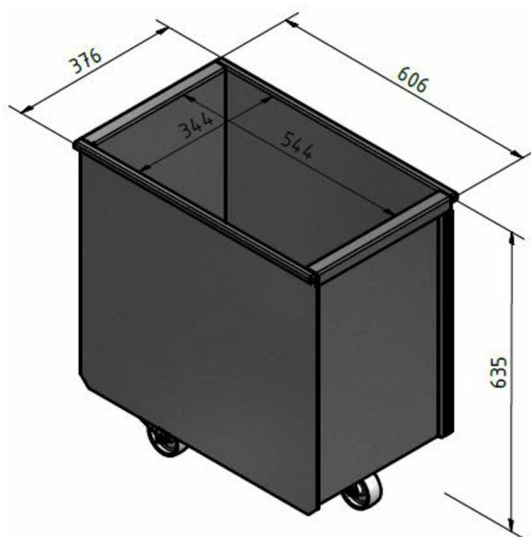
100 litrů Sběrná nádoba s kolečky
