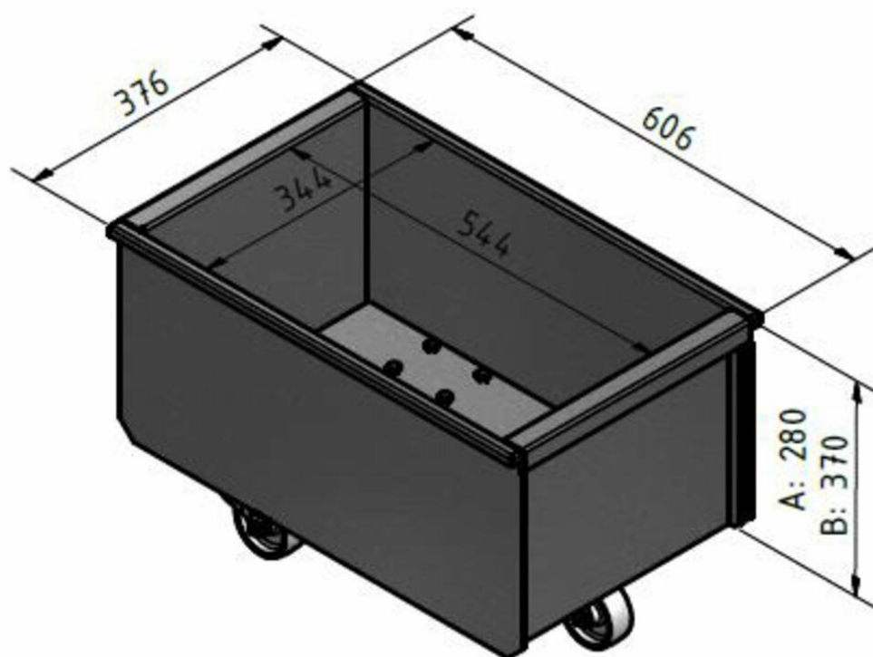
50 litrů Sběrná nádoba bez koleček (A) Sběrná nádoba s kolečky (B)
