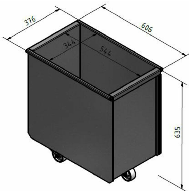
100 l Zbiornik do opróżniania z kółkami
