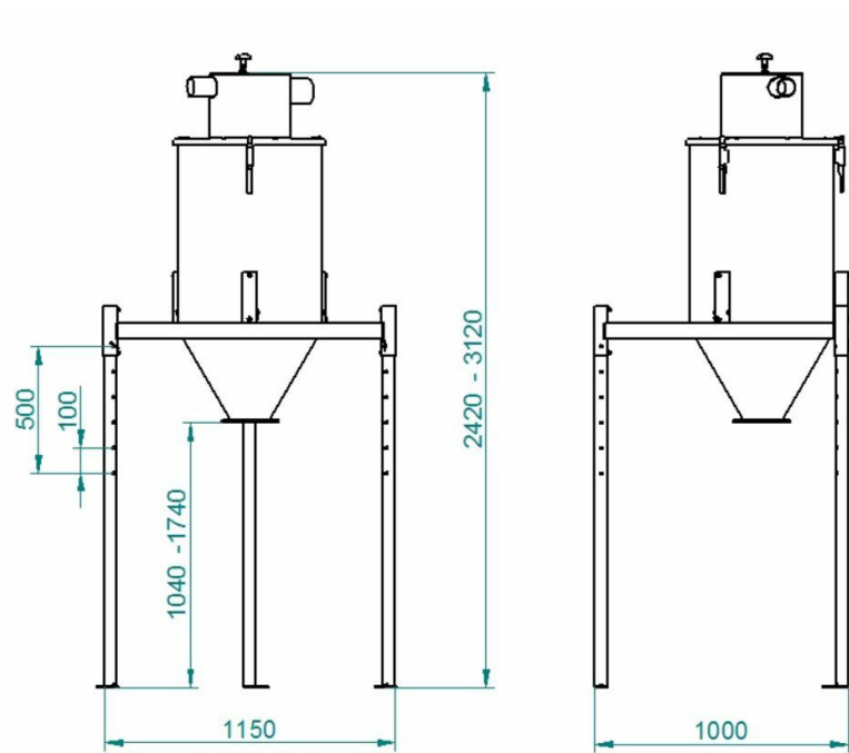
Abmessungen - Vorabscheidereinheit
