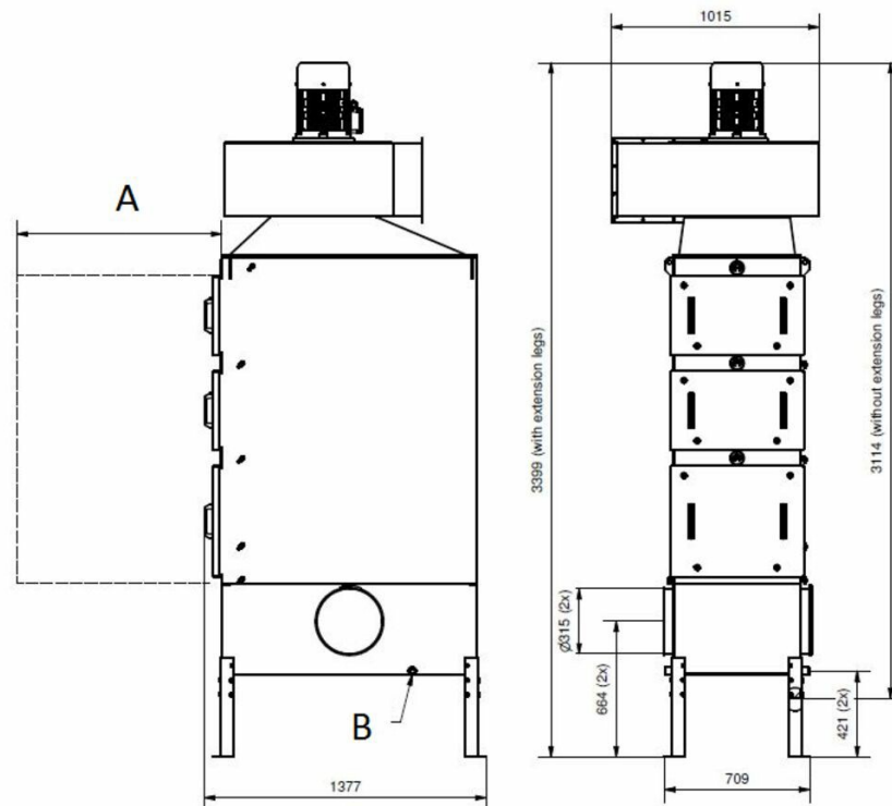
A) Espace de service minimum de 1000 mm B) Drainage DN25 (x2)
