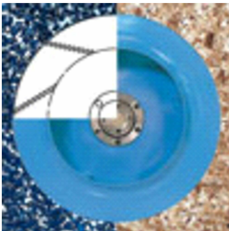
碎片叶轮 - S型 碎片叶轮是一个封闭、部分自清洁的叶片叶轮，带有直的后斜叶片。该叶轮用于输送打磨和抛光粉尘、干锯屑和切屑等。碎片叶轮的效率最高81%。
