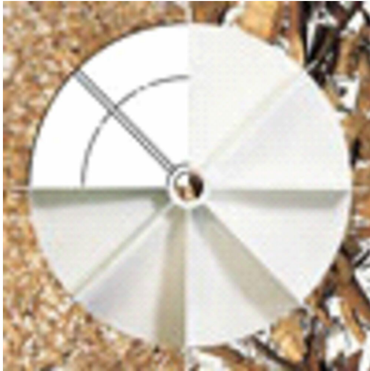
输送叶轮 - T型 输送叶轮是开放、自清洁叶片叶轮，带直的径向叶片。该叶轮用于输送切屑、碎片等。输送叶轮的效率最高61%。
